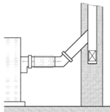
Figura 10. Tiro de chimenea.
