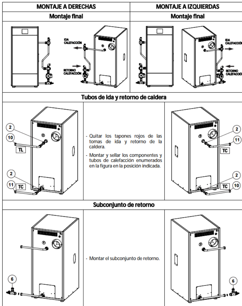
Esquema 5. Kit de circulación 2.
