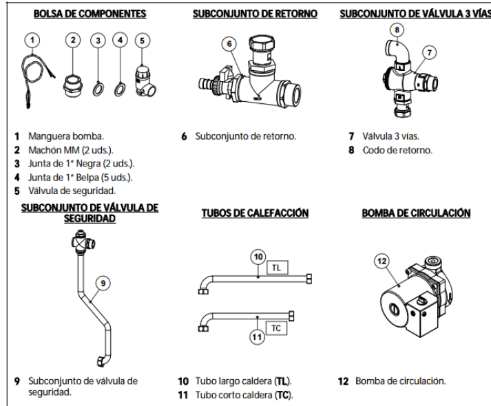
Esquema 4. Kit de circulación 1.
