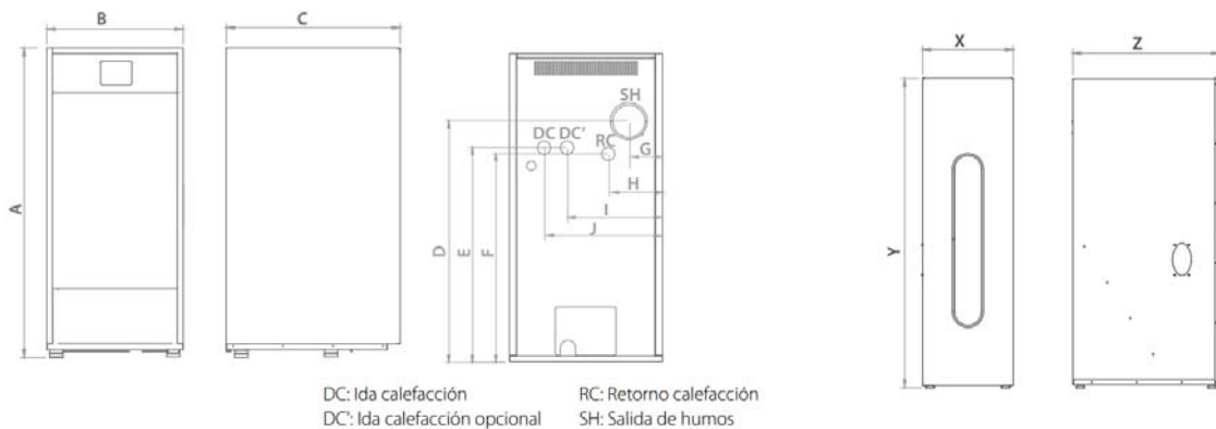
Figura 3. Dimensiones de Calderas y silo.
