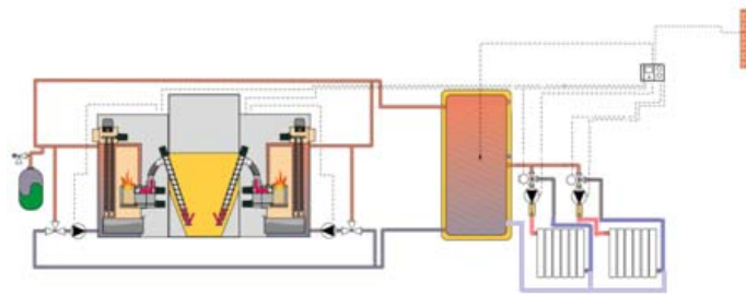
Esquema 3. Hidráulica de sistema de dos calderas en cascada.
