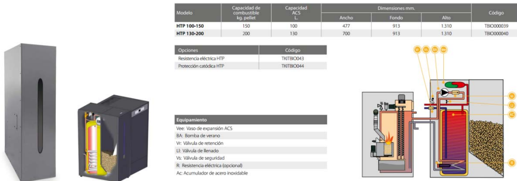
Figura 6. Depósito de acumulación.
