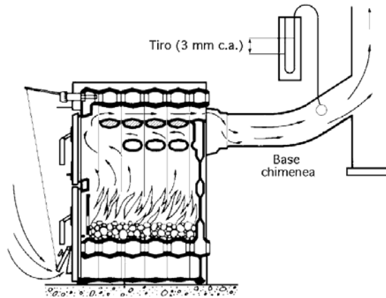
Figura 9. Funcionamiento de caldera de biomasa.
