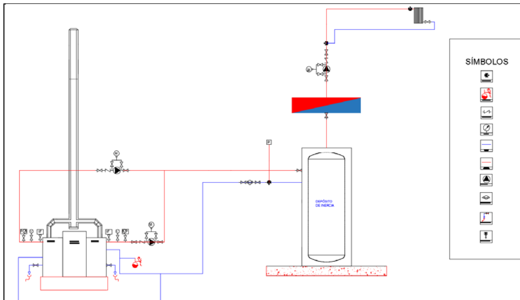
Esquema 7. Hidráulico de caldera doble de Pellets y Huesos de Aceitunas.
