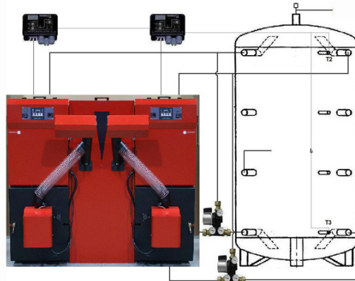
Esquema 2. Grupo térmico Caldera doble.
