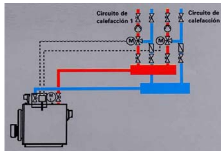
Esquema 1. Hidráulica de sistema de Gasóleo de Colegio Público de Calaceite.
