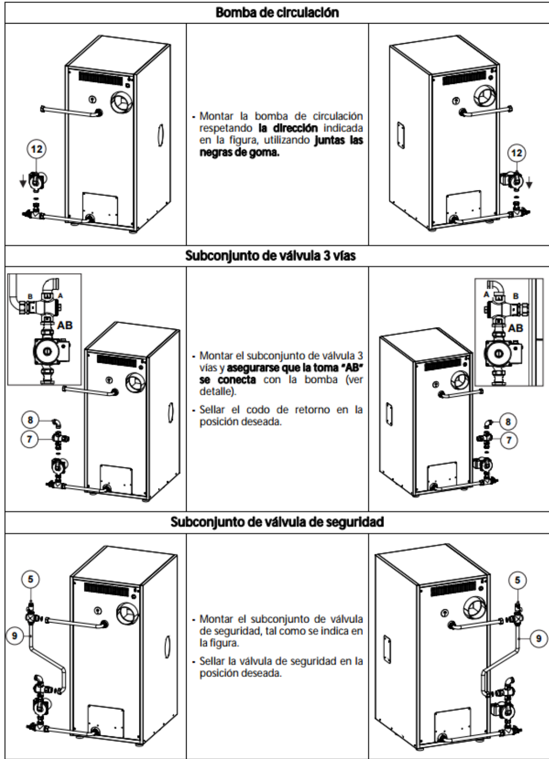
Esquema 6. Bomba de circulación.
