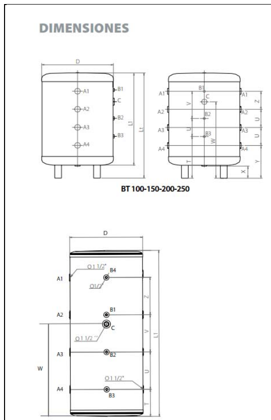
Figura 7. Depósito de Inercia.
