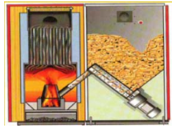
Figura 2. Caldera de Pellets y Huesos de aceituna.
