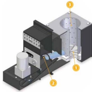
Figura 5. Quemador autolimpiable.
